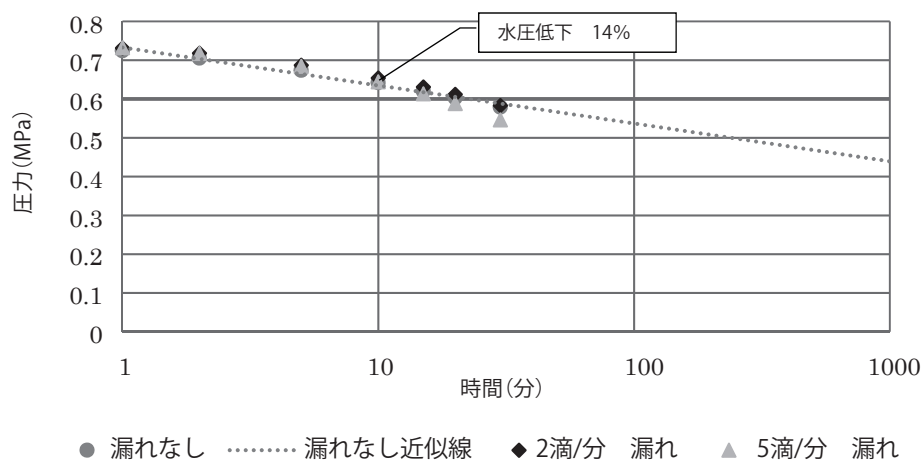
図 19 1 種二層管(PE50) 呼び径 50
