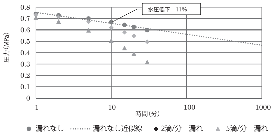
図 22 3 種二層管(PE100) 公称外径 32
