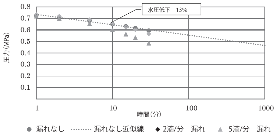
図 23 3 種二層管(PE100) 公称外径 40
