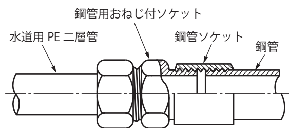
図20 鋼管との接続(おねじ)
