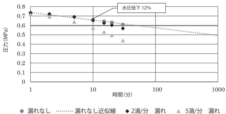
図 18 1 種二層管(PE50) 呼び径 25
