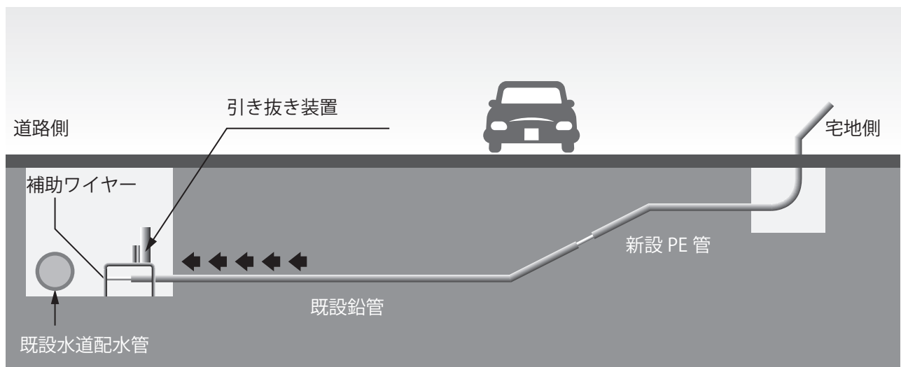
図 24 非開削工法のイメージ
