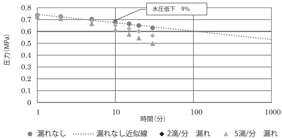
図 21 1 種二層管(PE100) 呼び径 40
