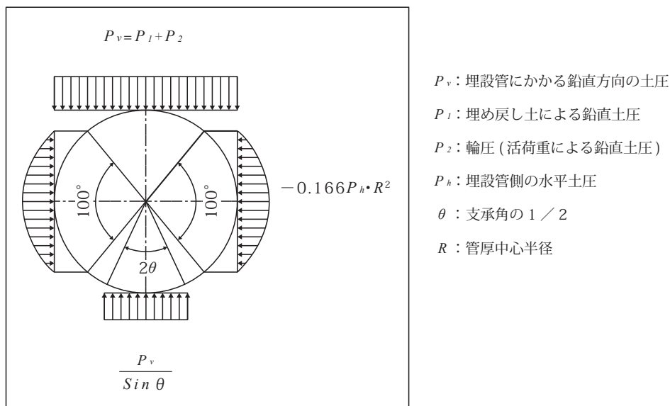
図 7 スパングレーの土圧分布図
