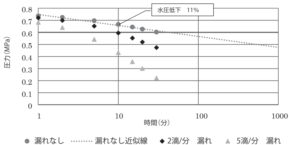
図 20 1 種二層管(PE100) 呼び径 25
