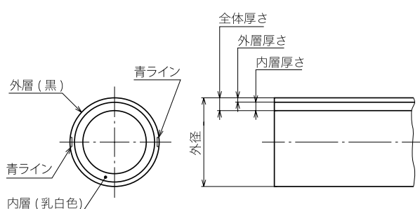
図 1 - 管の構造及び色 (3 種二層管公称外径 25 ～ 50)
