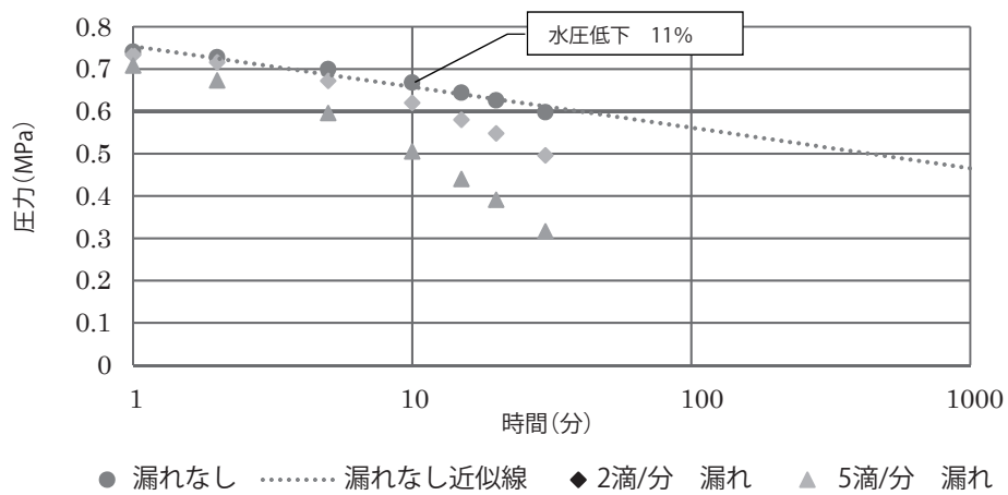
図 38 3 種二層管(PE100) 公称外径 32
