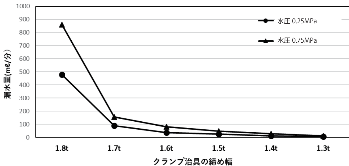
図10 クランプ治具の締め幅と通水量（漏水量）の関係（1 種二層管 PE50 呼び径 50）
