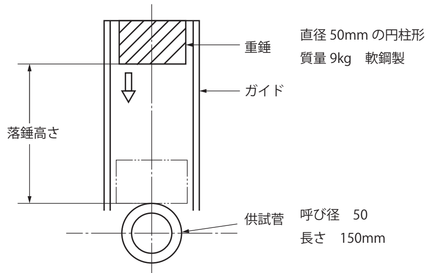
図 6 落錘式衝撃試験法
