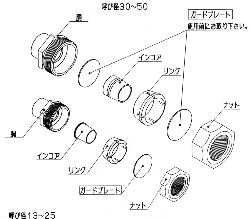
図 15 JWWA B 116 の各部品名称
