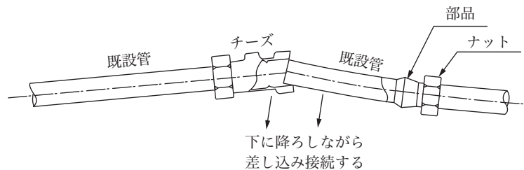
図34 おがみあわせ接続(チーズ)
