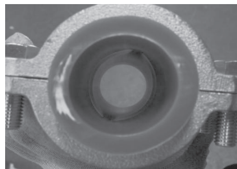
図 22 スクイズ部の管内面写真 (青色単層管(PE100) 呼び径 40)
