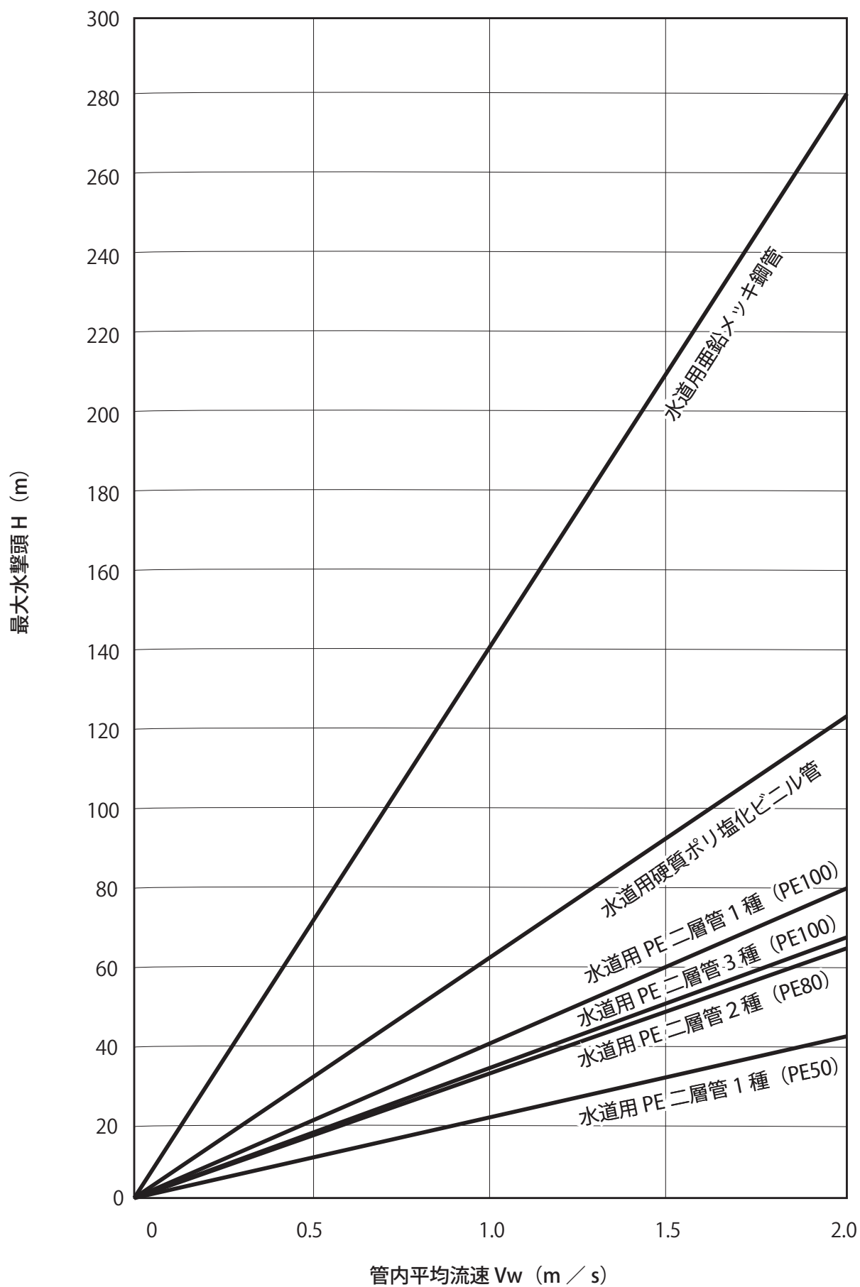
図5 各管種の水撃圧(呼び径25) ※水道用PE二層管3種は公称外径32
