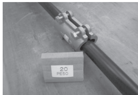
図 15 補修継手の取付確認 (1 種二層管 (PE50) 呼び径 20)
