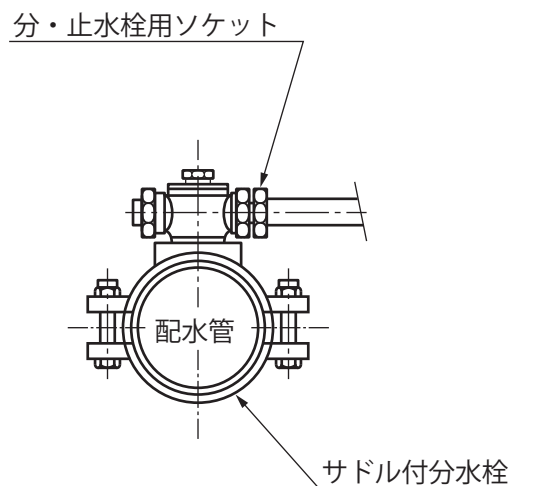
図 25 サドル付分水栓との接合
