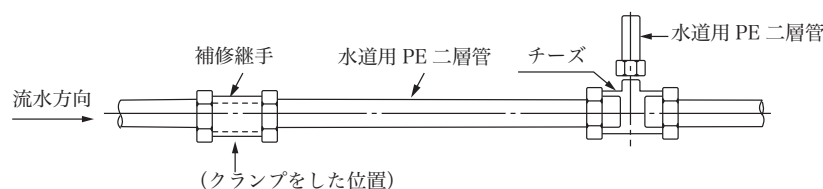
図6 分岐完成
