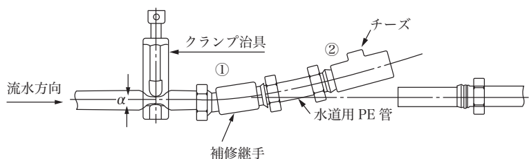
図5 継手挿入手順
