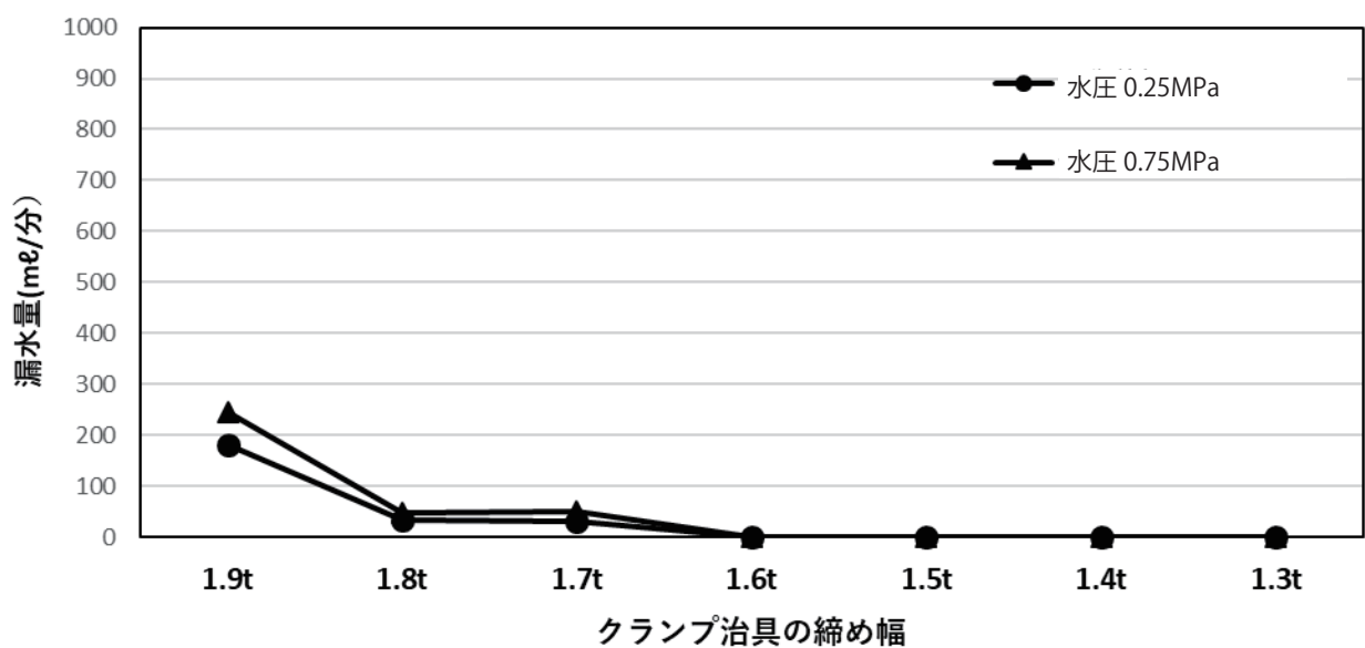
図 14 クランプ治具の締め幅と通水量(漏水量)の関係 (3 種二層管公称外径 50)
