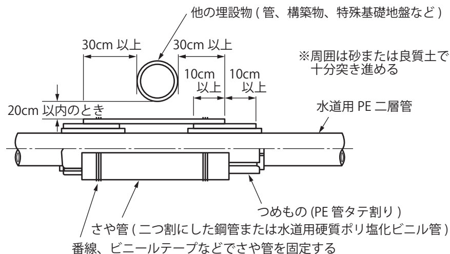
図 30 水道用 PE 二層管保護方法（水道用 PE 二層管を布設済の場合）
