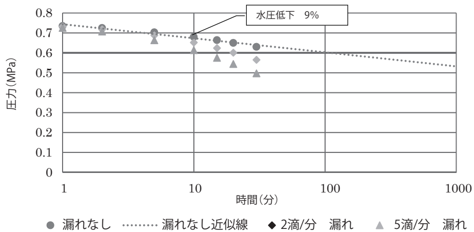
図 37 1 種二層管(PE100) 呼び径 40
