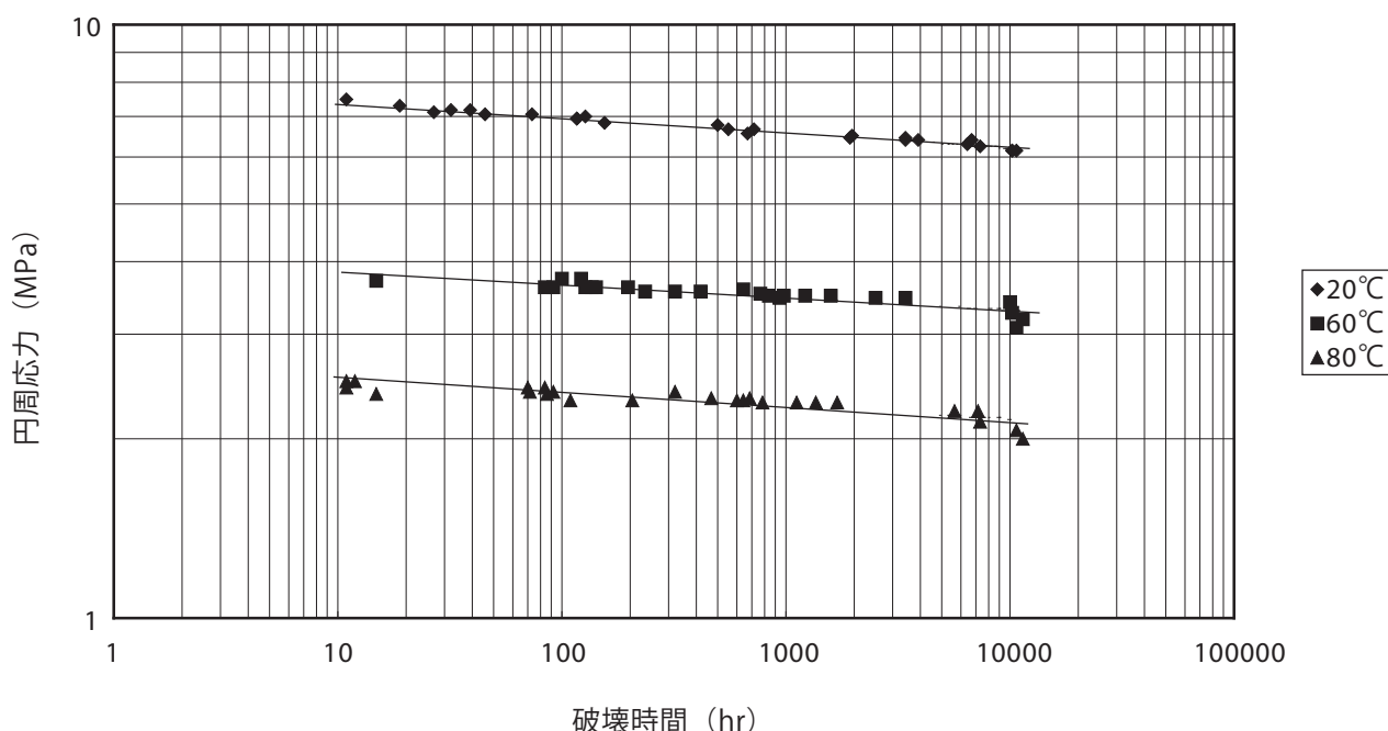
図 4 長期内圧クリープ線図
