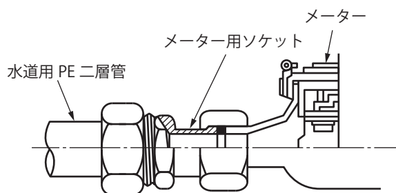
図 23 メーターとの接合
