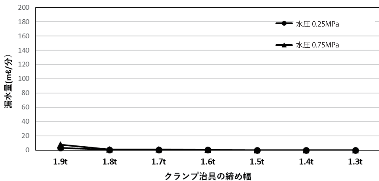
図 13 クランプ治具の締め幅と通水量(漏水量)の関係 (3 種二層管公称外径 25)
