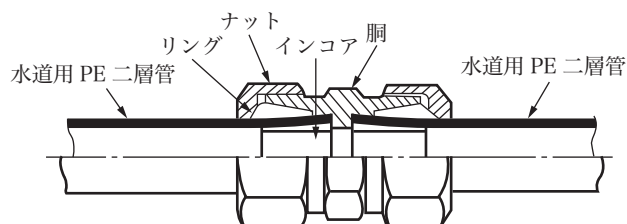
図14 冷間継手(JWWA B 116)
