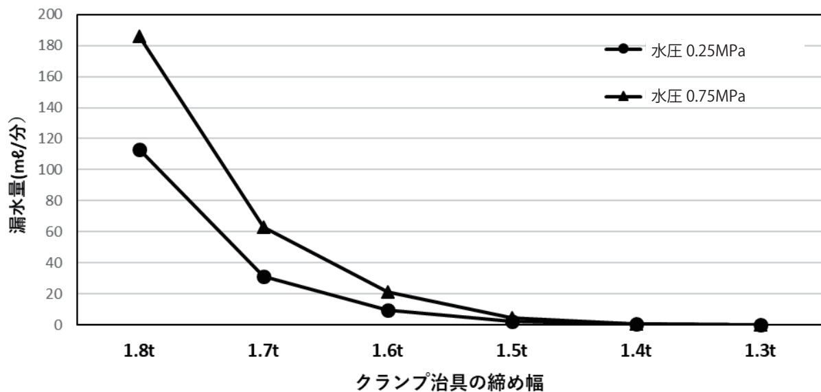
図9 クランプ治具の締め幅と通水量（漏水量）の関係（1 種二層管 PE50 呼び径 20）
