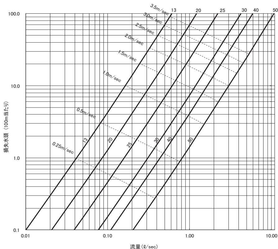
図 10-1 水道用 PE 二層管（1 種二層管（PE50、PE100 共通））
