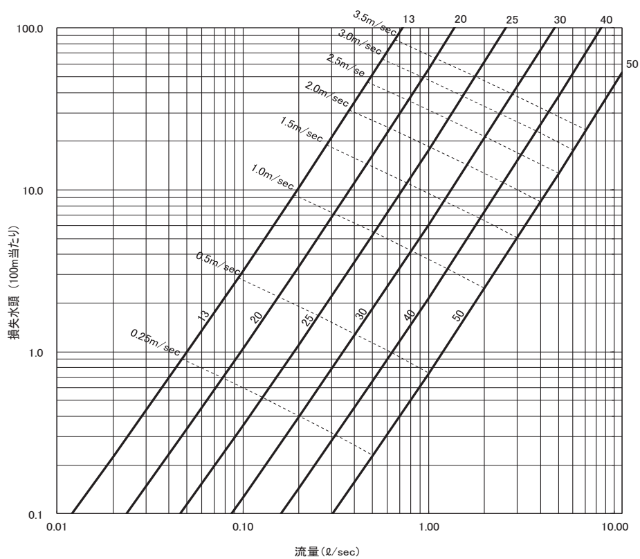
図 10-3 水道用 PE 二層管 (3 種二層管)
