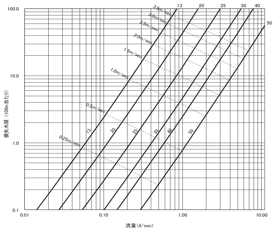
図 10-2 水道用 PE 二層管 (2 種二層管)
