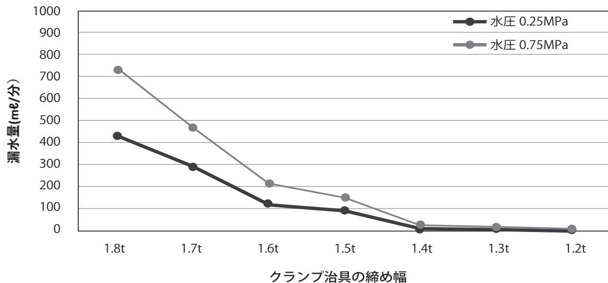
図 12 クランプ治具の締め幅と通水量(漏水量)の関係 (1 種二層管 PE100 呼び径 40)
