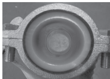
図 19 スクイズ部の管内面写真 (1 種二層管 (PE50) 呼び径 40)
