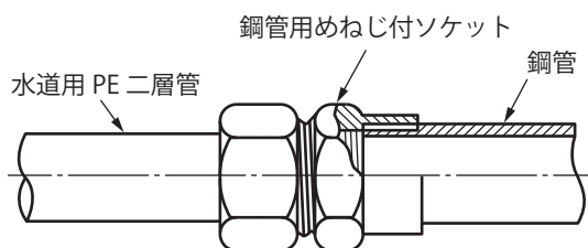
図19 鋼管との接続(めねじ)
