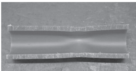
図 25 スクイズ部の内面 全体と拡大（1 種二層管 (PE50) 呼び径 40)
