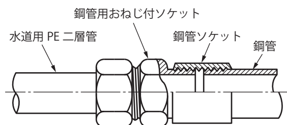
図20 鋼管との接続(おねじ)
