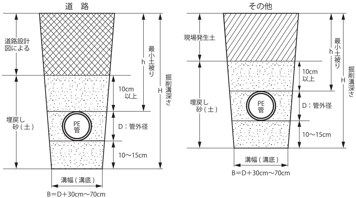
図28 水道用PE二層管の標準埋め戻し断面
