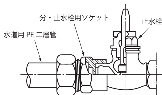
図 24 止水栓との接合
