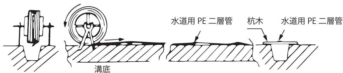
図 32 呼び径 25 以下の長尺配管要領
