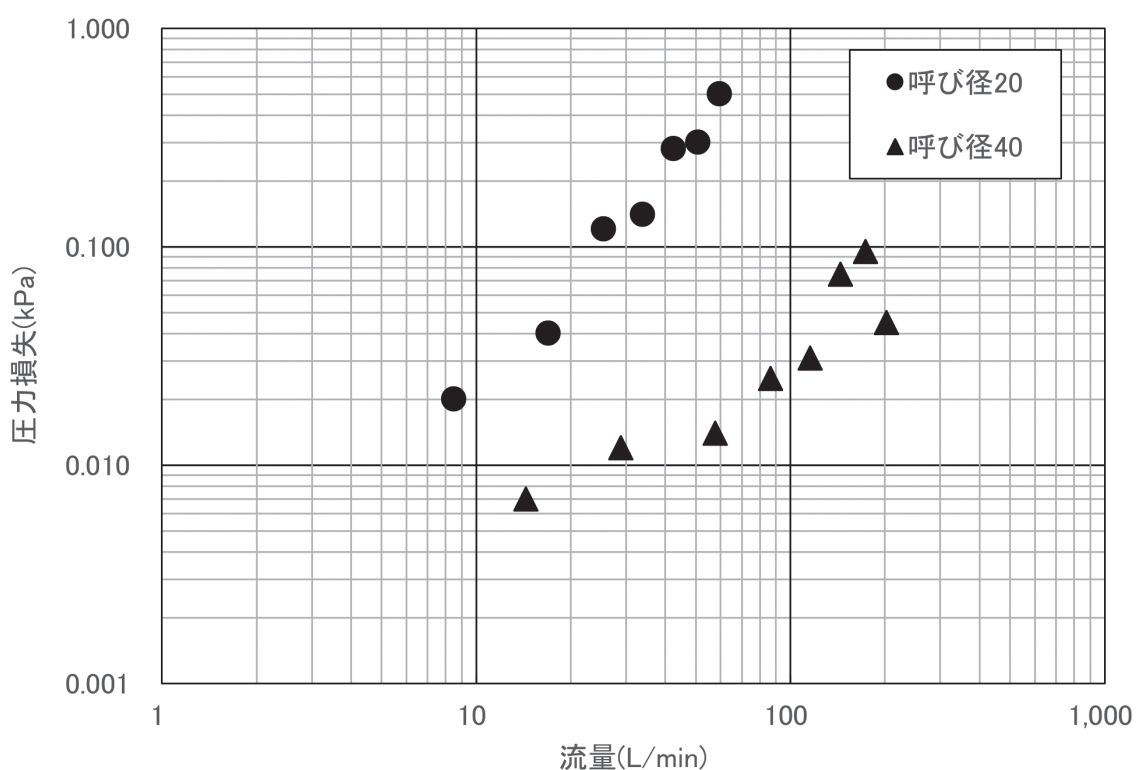
図 17 圧力損失の測定結果 (1種二層管(PE50))
