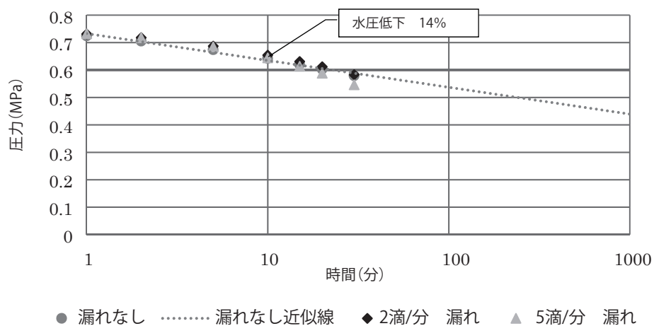
図 35 1 種二層管(PE50) 呼び径 50
