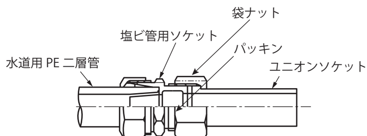
図 21 硬質ポリ塩化ビニル管との接合
