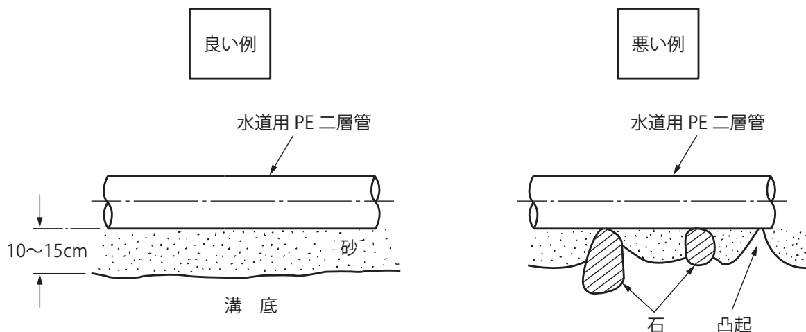
図27 溝床仕上げ例
