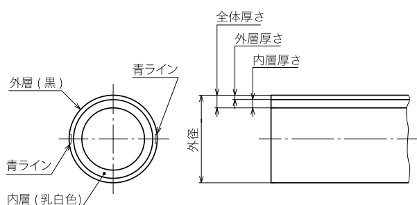
図 1 - 管の構造及び色 (3 種二層管公称外径 25 ~ 50)
