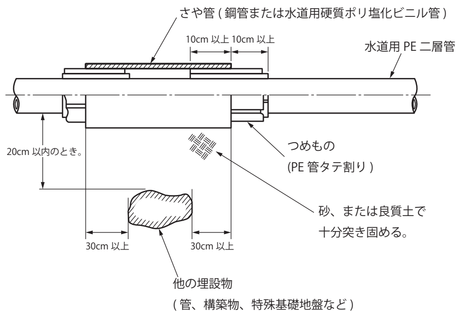
図 29 水道用 PE 二層管保護方法（水道用 PE 二層管を新設する場合）
