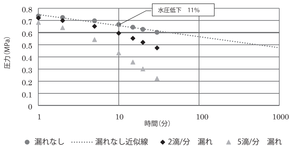
図 36 1 種二層管(PE100) 呼び径 25
