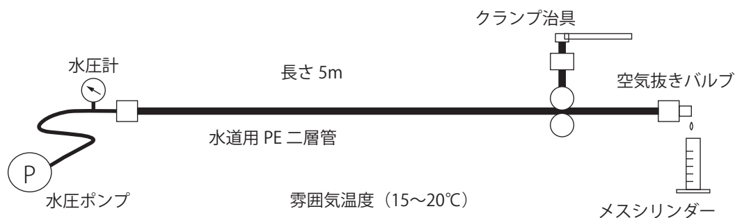
図8 実験配管状況
