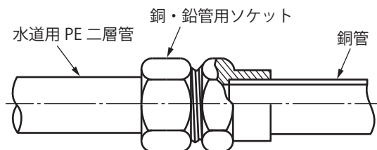
図 22 銅管との接合
