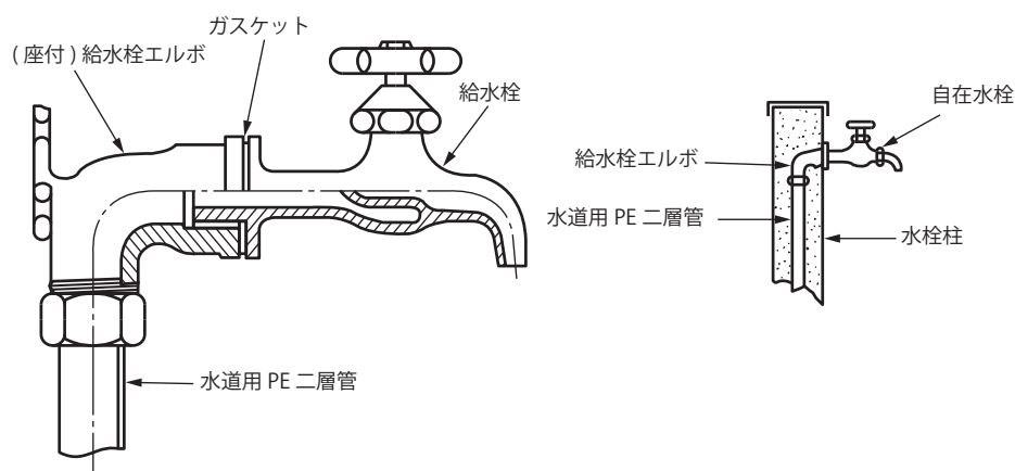
図26 給水栓との接合
