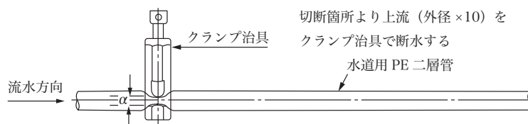
図4 クランプ治具による断水
