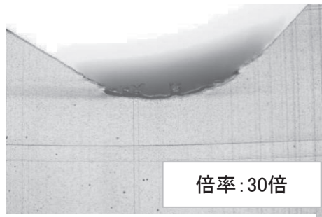
図 24 スクイズ部の断面 全体と拡大（1 種二層管 (PE50) 呼び径 20)
