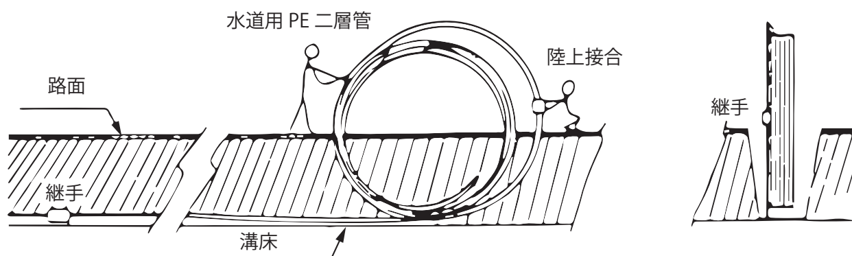
図 33 呼び径 30 以上の長尺配管要領
