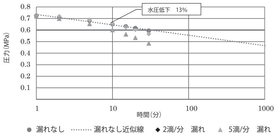
図 39 3 種二層管(PE100) 公称外径 40
