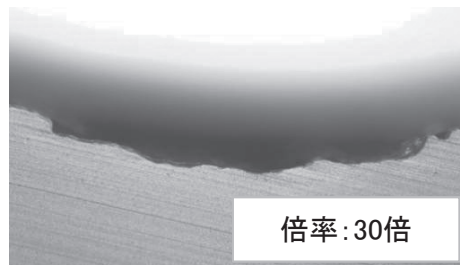
図 26 スクイズ部の断面 全体と拡大（1 種二層管 (PE50) 呼び径 40)
