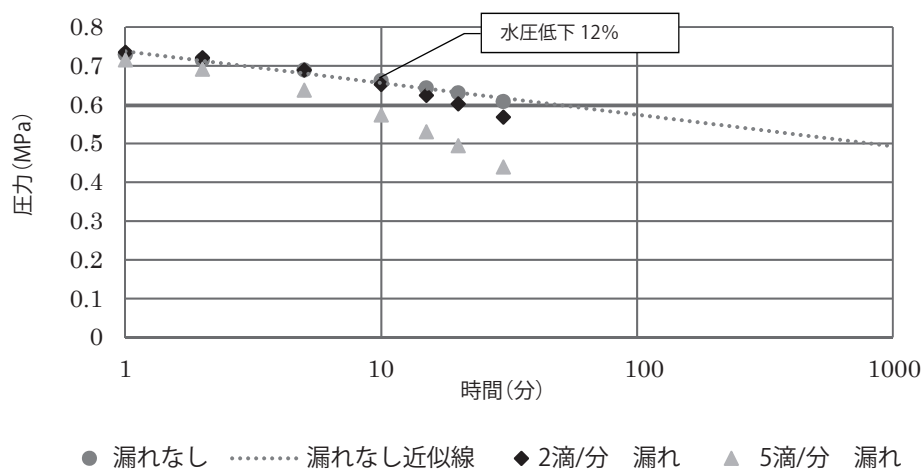
図 34 1 種二層管(PE50) 呼び径 25
