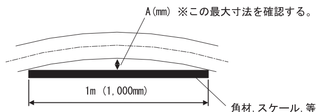
図31 最小曲げ半径の施工管理方法
