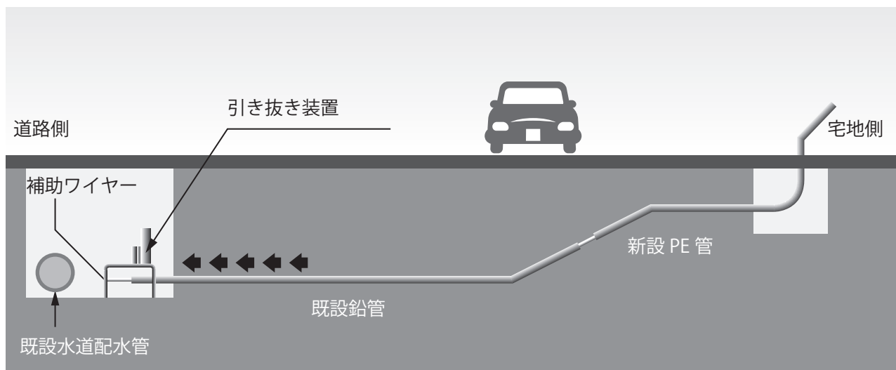
図 40 非開削工法のイメージ
