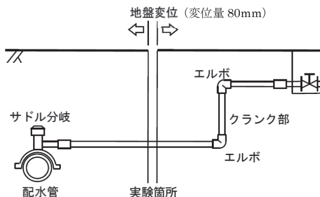
図 8 実験モデル
