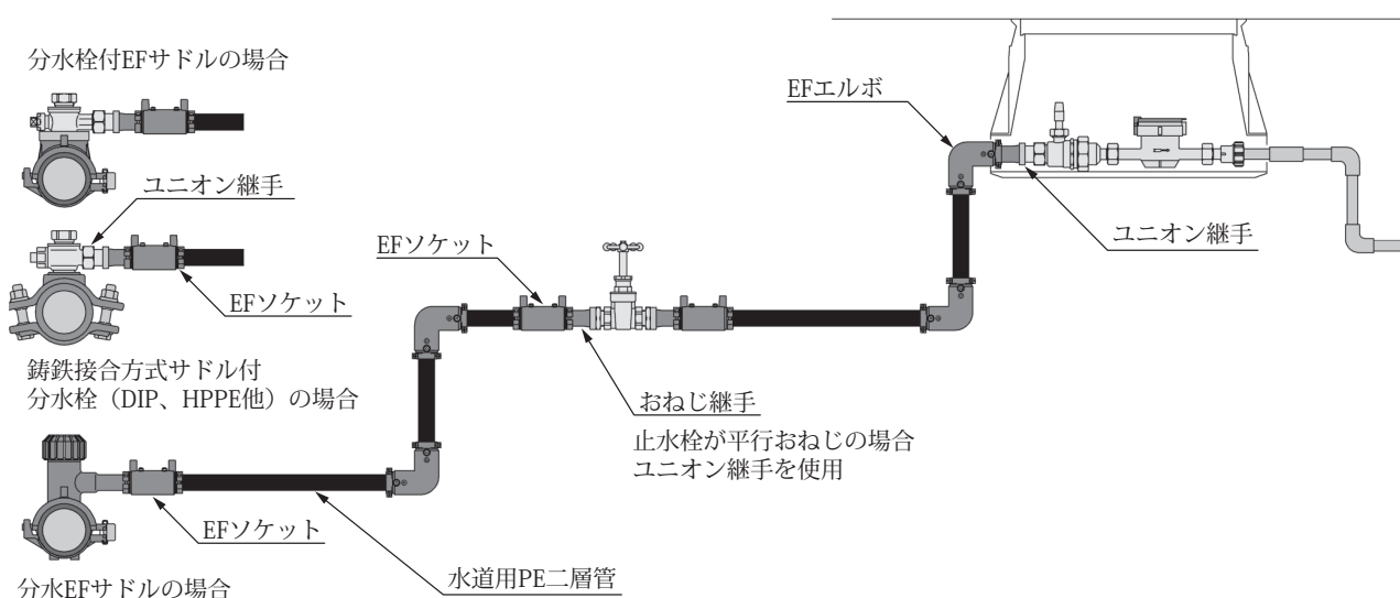
図 13 水道用 PE 二層管の配管例（EF 継手使用時）
