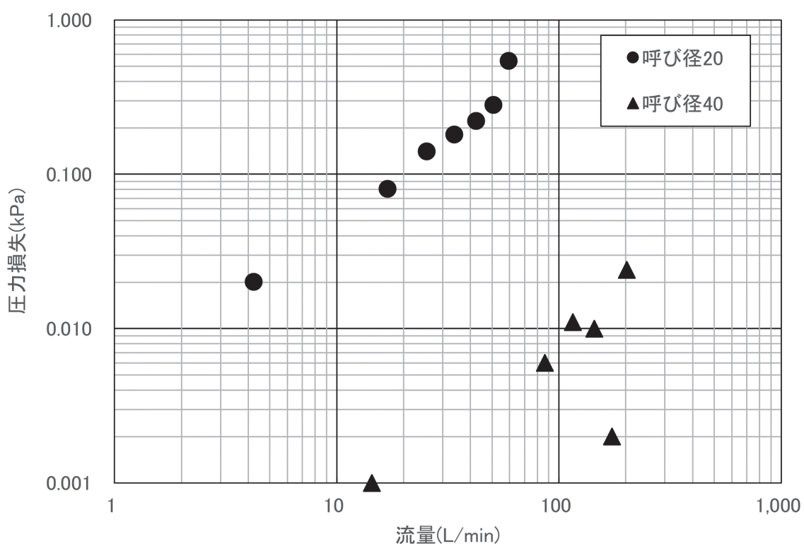
図 20 圧力損失の測定結果 (1 種二層管 (PE100))
