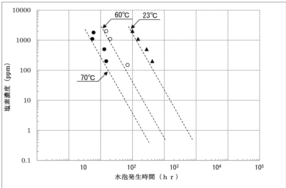
図2 1種単層管
