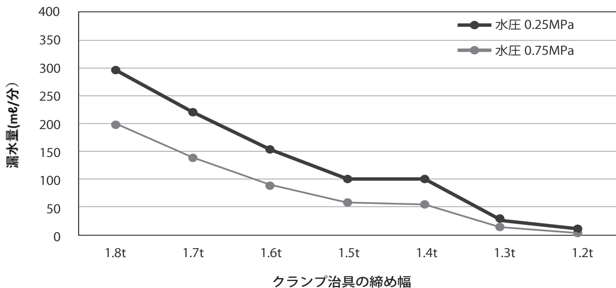
図11 クランプ治具の締め幅と通水量（漏水量）の関係（1 種二層管 PE100 呼び径 20）
