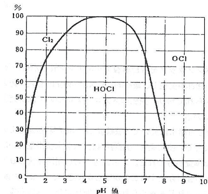
図1 水中遊離塩素の形に対する pH の影響
