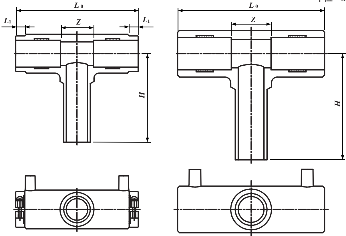
付表 4－EF チーズ
