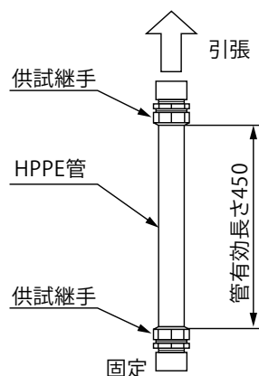
図 A2 ー高速引張試験装置
