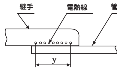
図4—はく離面の測定方法
