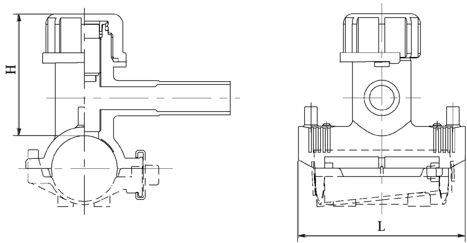
付表 12 ー止水機構付 EF サドル
