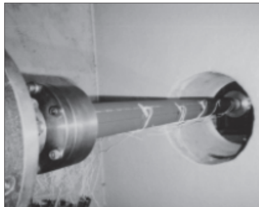
管軸方向引張り試験の状況
