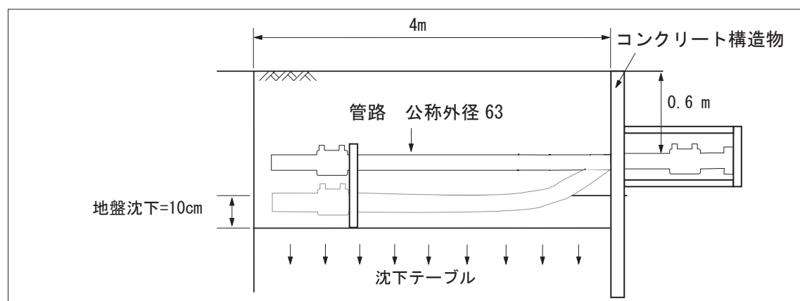
図-4.16 構造物際貫通部の段差沈下試験
