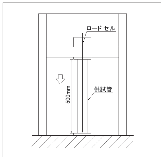
図-4.8 管軸方向圧縮試験
