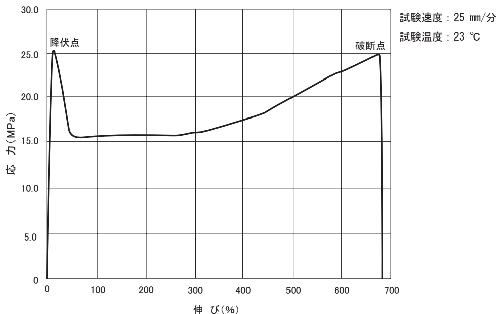
図-4.1 引張試験結果
