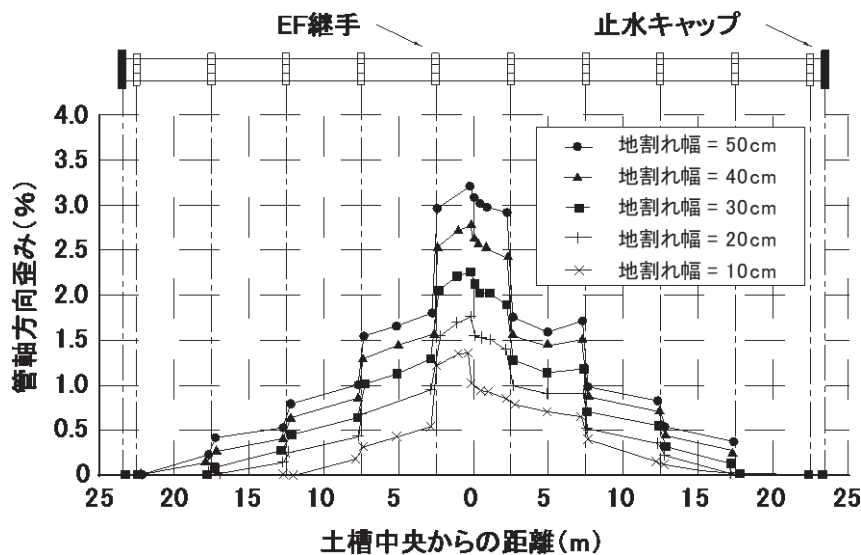
図-4.13 管軸方向歪み分布
