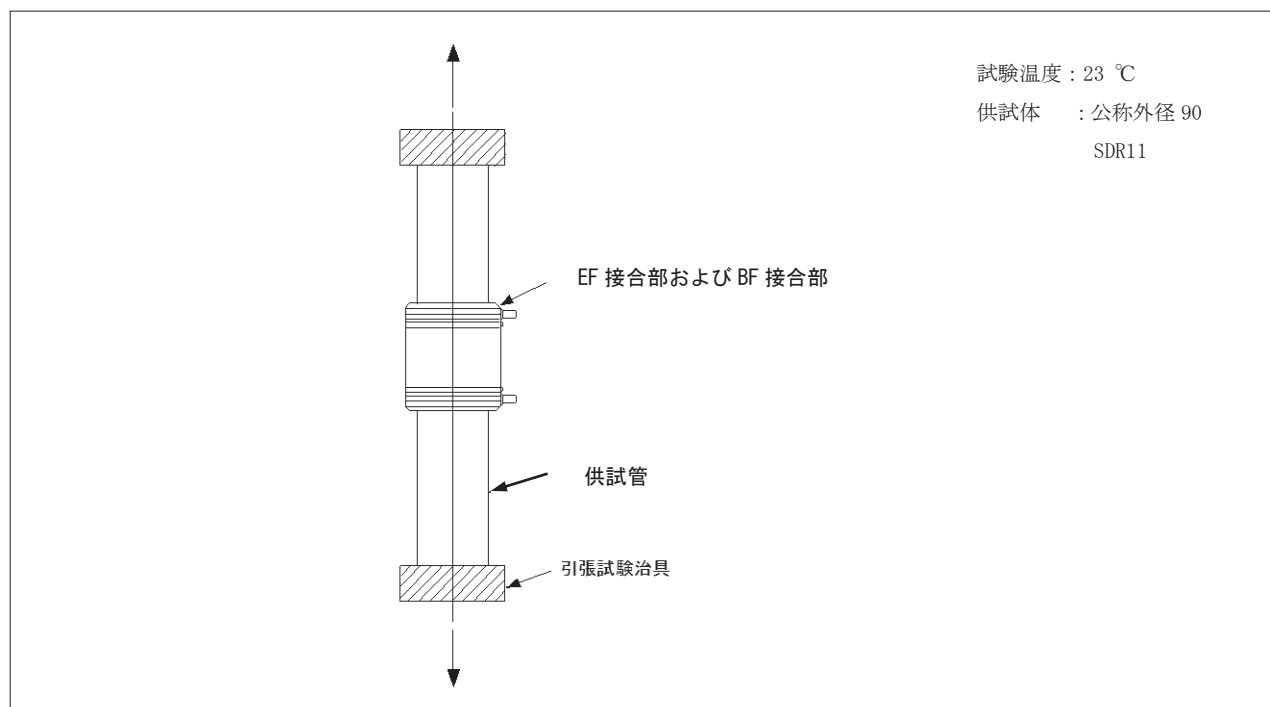
図-4.3 引張試験
