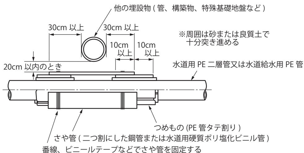
図 31 水道用 PE 二層管又は水道給水用 PE 管保護方法（水道用 PE 二層管又は水道給水用 PE 管を布設済の場合）
