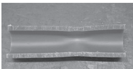
図 29 スクイズ部の内面 全体と拡大 (1種単層管(PE100) 呼び径40)
