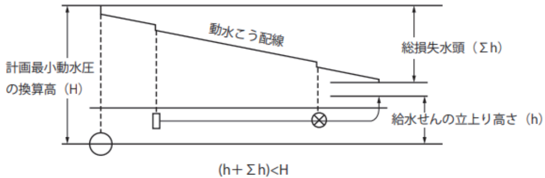
図 12 管径決定基準
