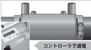
管と継手のセット・通電開始 電熱線が発熱を始め、樹脂の温度が上昇する。
