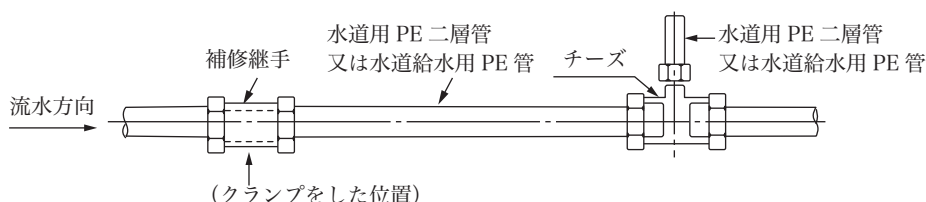
図6 分岐完成
