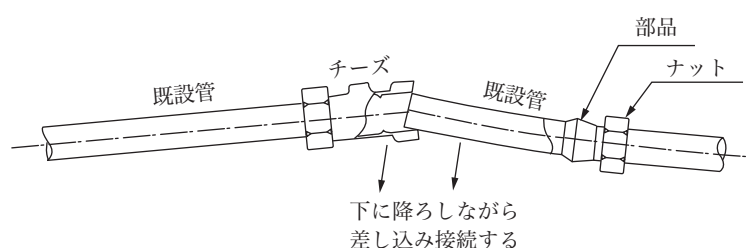
図35 おがみあわせ接続(チーズ)
