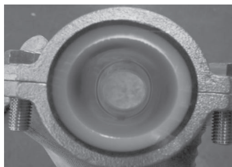
図 19 スクイズ部の管内面写真 (1種二層管(PE50) 呼び径 40)
