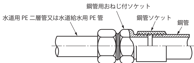
図21 鋼管との接続(おねじ)
