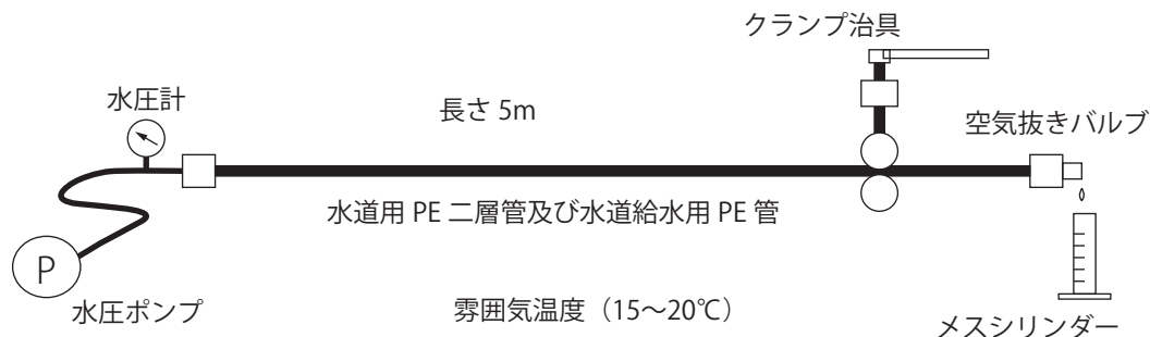
図8 実験配管状況
