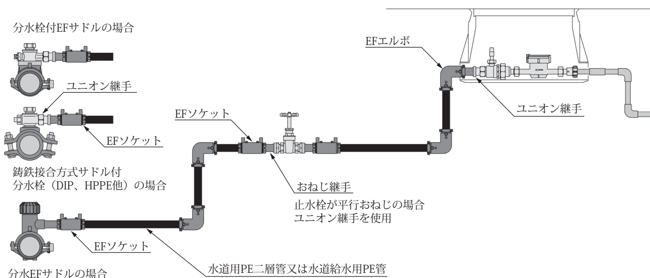
図 14 水道用 PE 二層管及び水道給水用 PE 管の配管例（EF 継手使用時）
