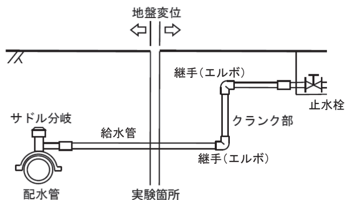
図8 実験モデル
