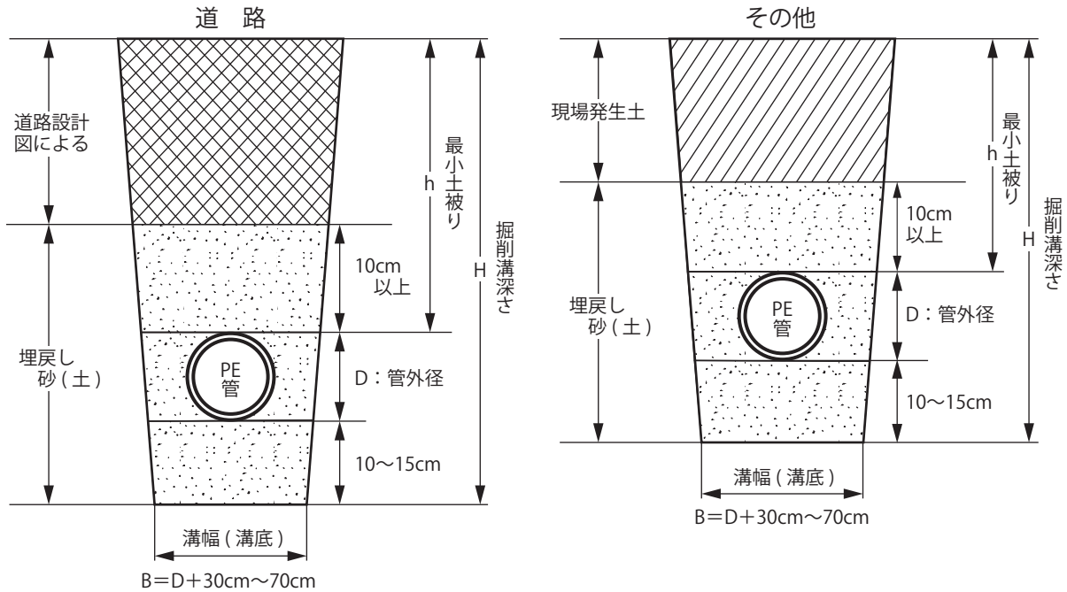
図29 水道用PE二層管又は水道給水用PE管の標準埋め戻し断面
