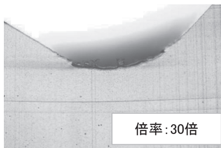
図 28 スクイズ部の断面 全体と拡大 (1種単層管(PE100) 呼び径 20)
