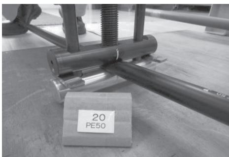
図 15 補修継手の取付確認 (1 種二層管 (PE50) 呼び径 20)
