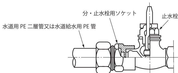
図 25 止水栓との接合
