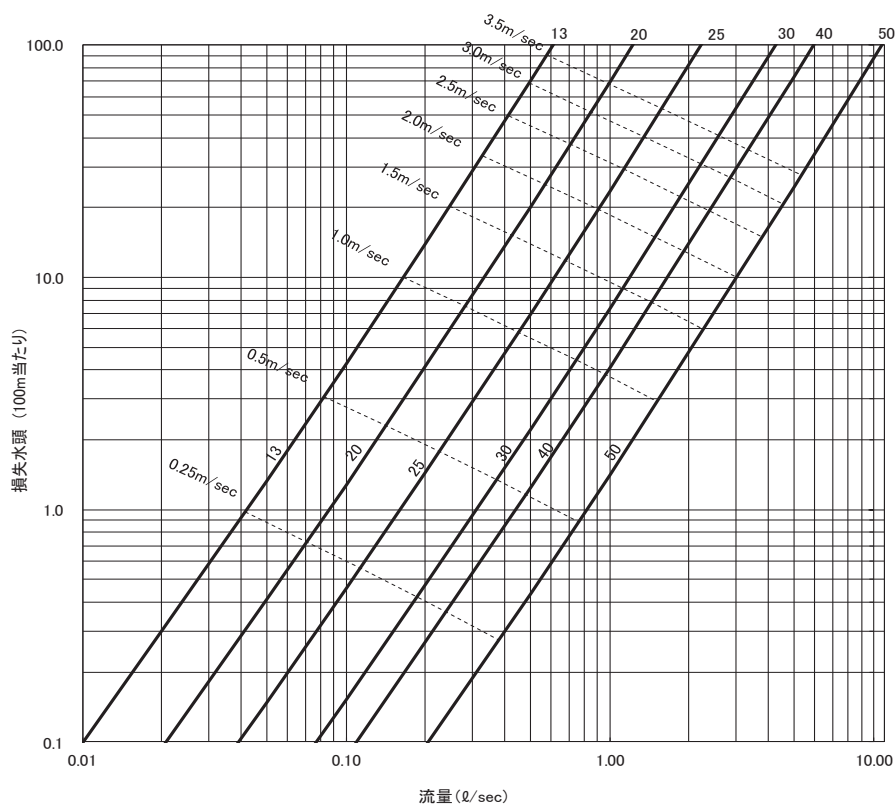
図 11-1 水道用 PE 二層管（1 種二層管（PE50、PE100 共通））、水道給水用 PE 管
