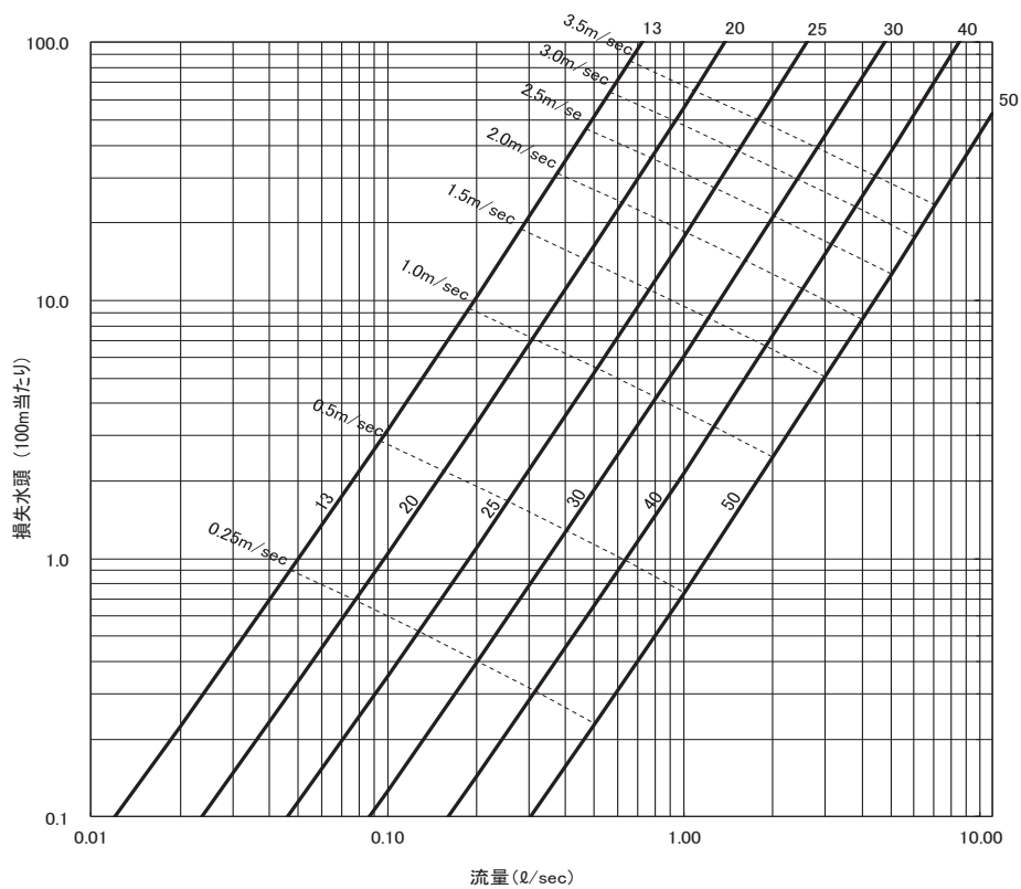
図 11-3 水道用 PE 二層管 (3 種二層管)
