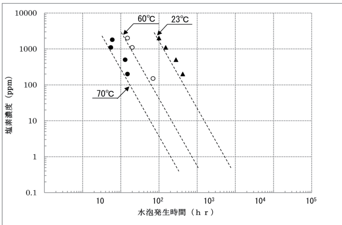
図2 1種単層管
