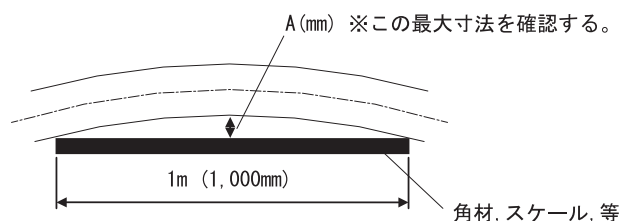
図32 最小曲げ半径の施工管理方法
