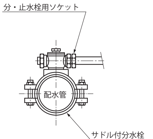
図 26 サドル付分水栓との接合
