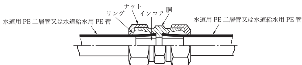
図15 金属継手(JWWA B 116)
