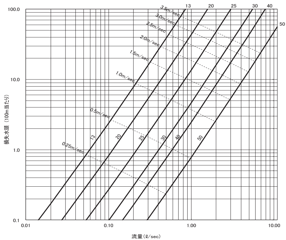
図 11-2 水道用 PE 二層管 (2 種二層管)
