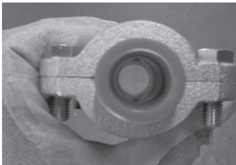
図 21 スクイズ部の管内面写真 (1種単層管 (PE100) 呼び径20)
