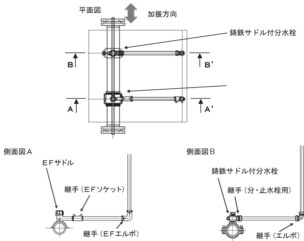
図10 実験モデル
