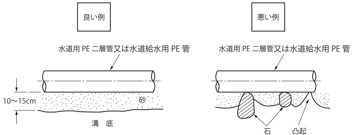
図28 溝床仕上げ例
