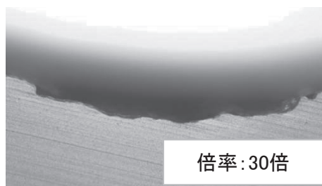
図 30 スクイズ部の断面 全体と拡大 (1種単層管(PE100) 呼び径40)
