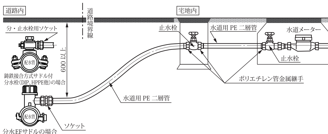
図 13 水道用 PE 二層管の配管例（金属継手使用時）
