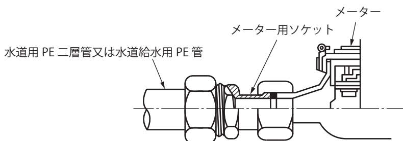
図 24 メーターとの接合
