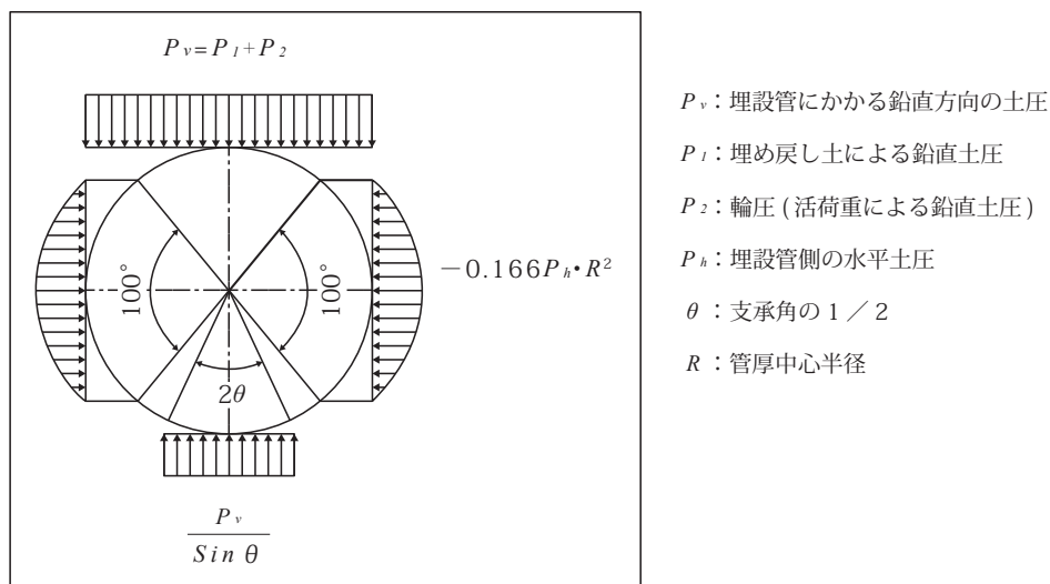
図 7 スパングラの土圧分布図
