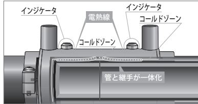
樹脂が加熱溶融されて膨張し、コールドゾーンで閉じ込められることにより、界面圧力が発生する。これにより管と継手の樹脂が融着されると同時にインジケータが押し上げられる。
