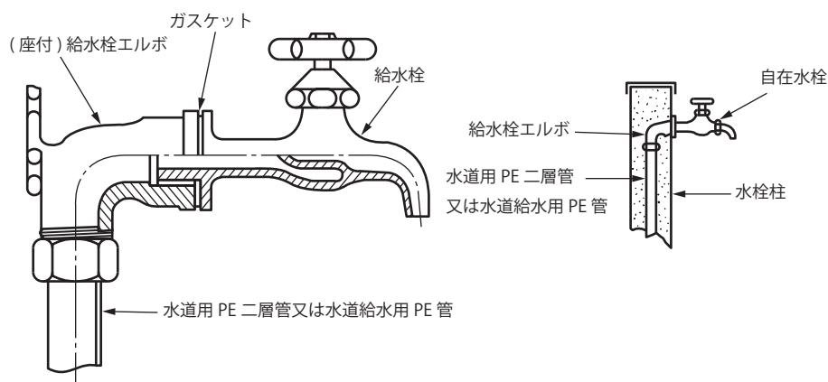
図27 給水栓との接合
