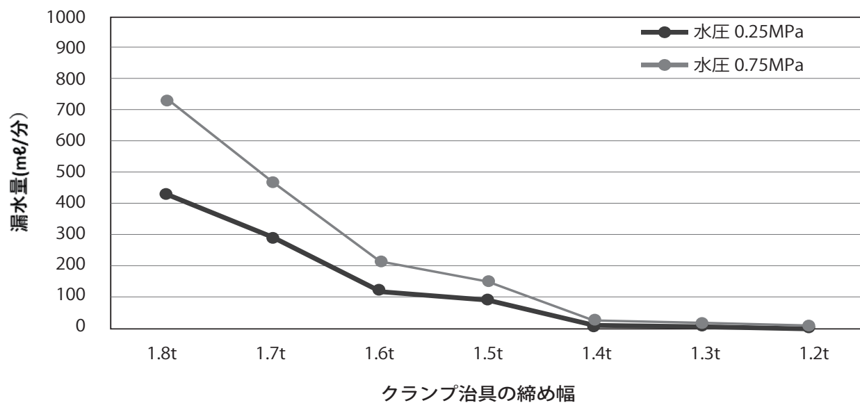
図 12 クランプ治具の締め幅と通水量(漏水量)の関係 (1 種単層管 PE100 呼び径 40)
