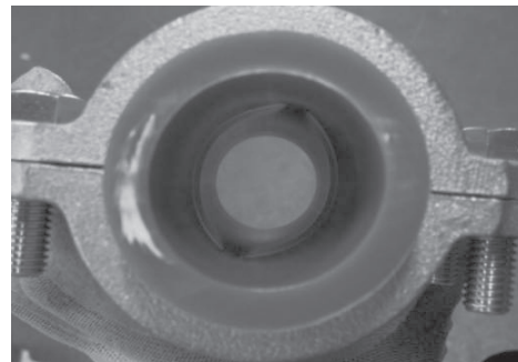
図 22 スクイズ部の管内面写真 (1種単層管 (PE100) 呼び径40)
