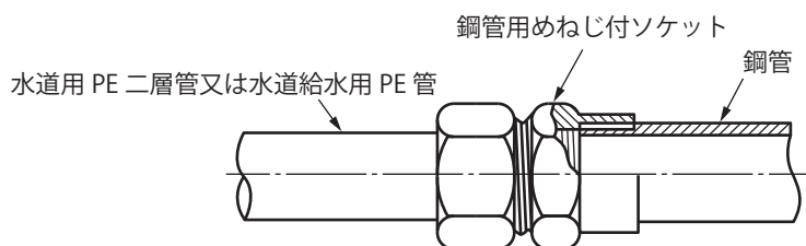
図20 鋼管との接続(めねじ)
