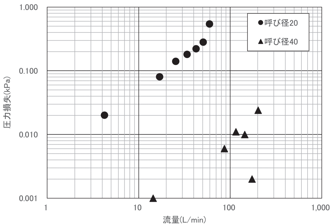
図 20 圧力損失の測定結果 (1種単層管 (PE100))
