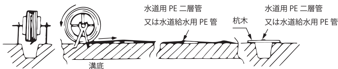
図 33 呼び径 25 以下の長尺配管要領
