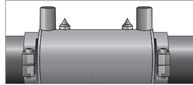
通電終了(自動)・冷却 溶融された樹脂が再び固化して融着が完了し、管と継手が組織的に一体化構造となる。
