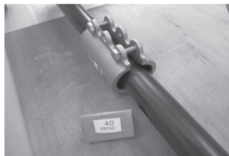
図 16 補修継手の取付確認 (1 種二層管 (PE50) 呼び径 40)
