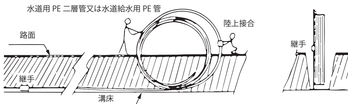
図 34 呼び径 30 以上の長尺配管要領
