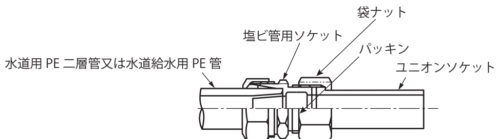
図 22 硬質ポリ塩化ビニル管との接合
