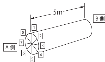
図7 管厚測定箇所
