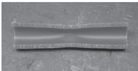
図 27 スクイズ部の内面 全体と拡大 (1種単層管(PE100) 呼び径20)
