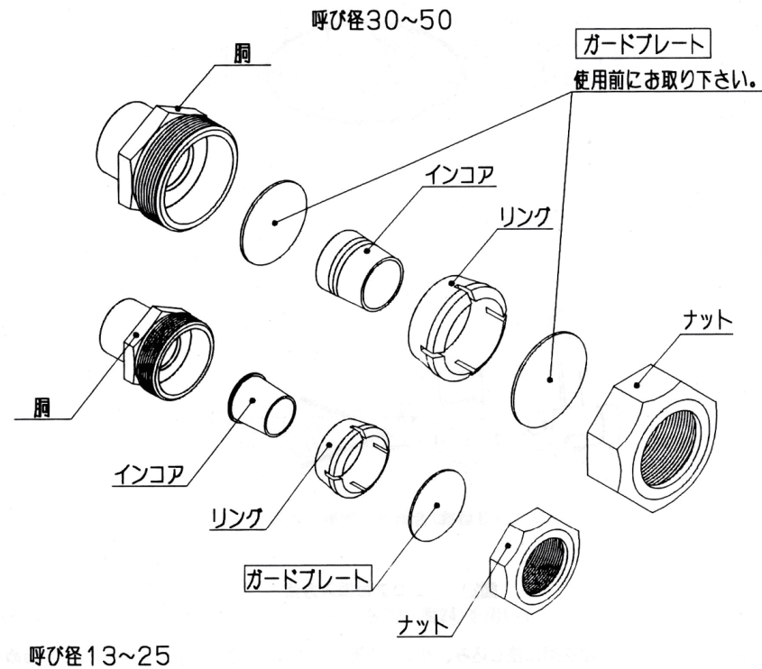
図 16 JWWA B 116 の各部品名称
