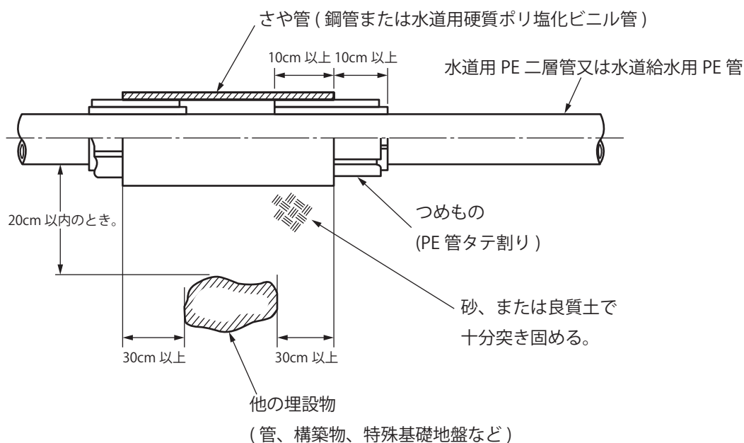
図 30 水道用 PE 二層管又は水道給水用 PE 管保護方法（水道用 PE 二層管又は水道給水用 PE 管を新設する場合）
