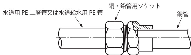
図 23 銅管との接合
